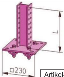
Ständerkonsole für Klemmanschluss Anschlussprofil 80 - 120 mm STL-SKK-
