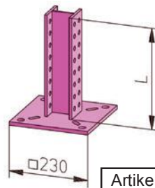
Ständerkonsole für Dübelanschluss Dübelplatte 230 x 230 x 10 mm STL-SKD-
